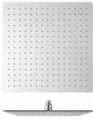
Kopfbrause Plus, quadratisch 400 × 400 mm, verchromt Art.-Nr. KB+SWP400E | 1.152,- €
